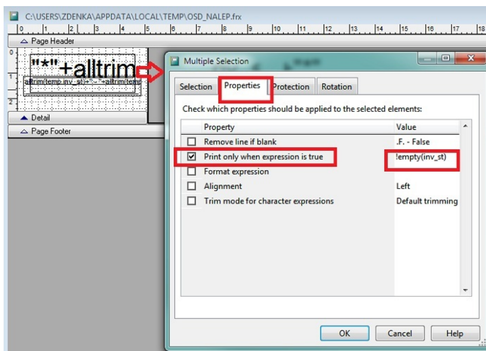
Slika: Uporabniška prilagoditev izpisa osd_nalep.*, pogoj ne zavihek Properties/Print only when
