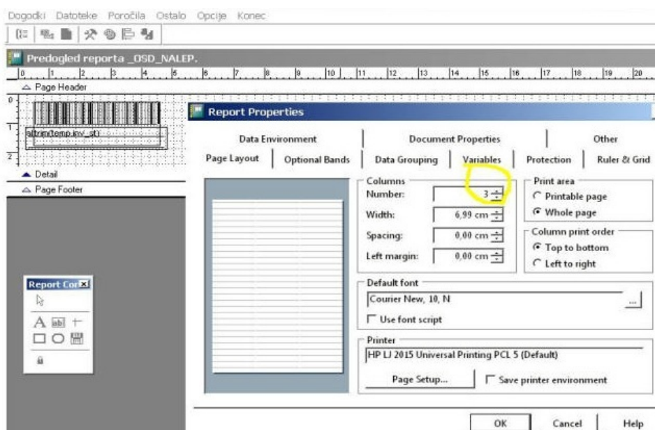
Slika: Uporabniška prilagoditev izpisa osd_nalep.*, sprememba števila nalepk v vrsti
